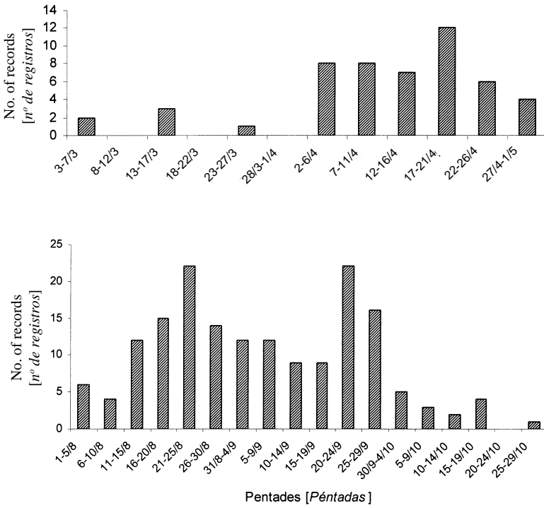
FIG. 3.—Aquatic Warbler Acrocephalus paludicola phenology between 1965 and 1998 in Spain based on ringing and observational data. [Fenología del Carricerín Cejudo Acrocephalus paludicola entre 1965 y 1998 en España, basada en datos de anillamiento y observaciones.]
