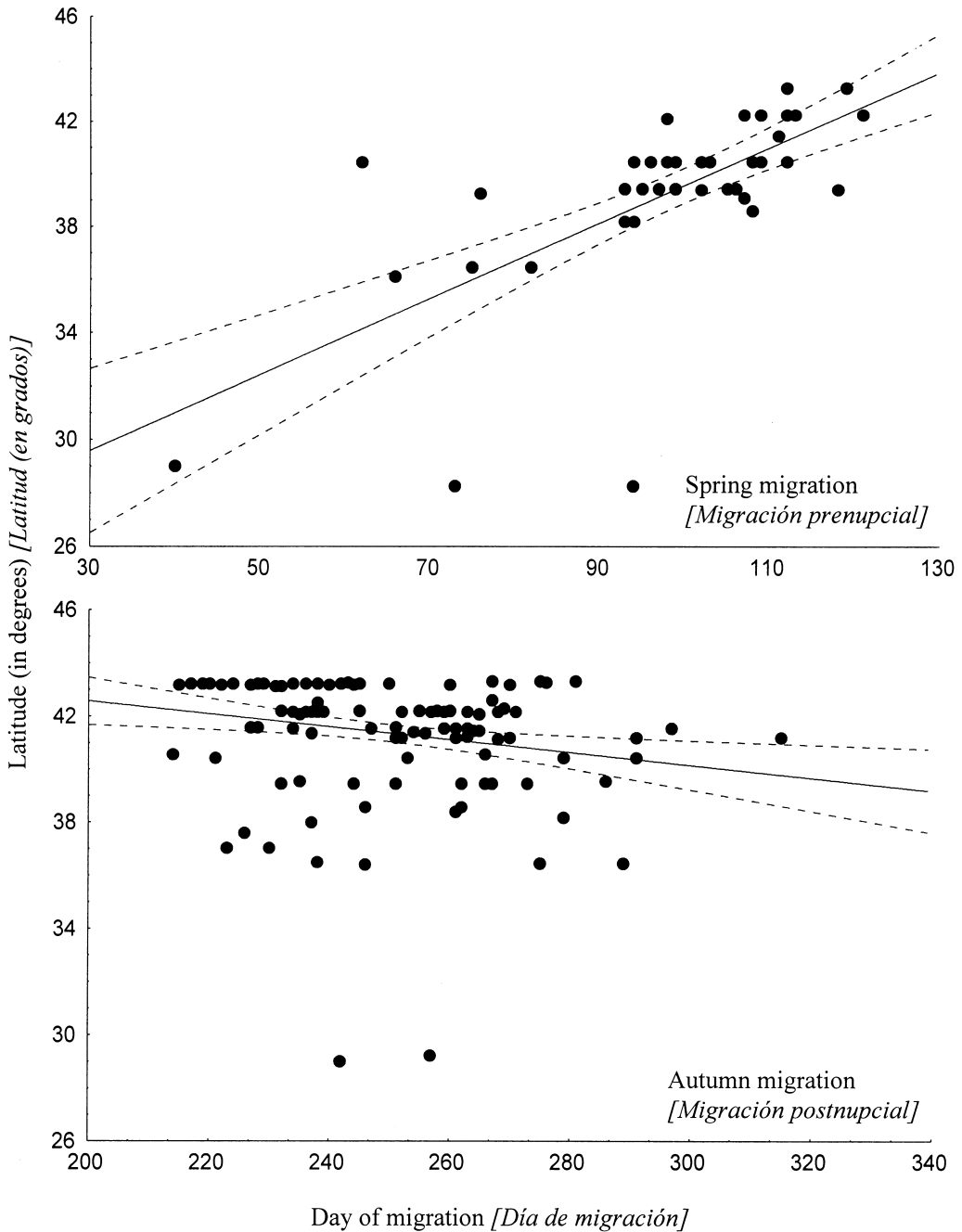
FIG. 4.—Relationship between day of migration of Aquatic Warbler Acrocephalus paludicola in Spain and latitude (in degrees). Date of migration is displayed according to Julian Calendar (1 Jan = 1; 31 Dec = 365). [Relación entre el día de migración del Carricerín Cejudo Acrocephalus paludicola en España y la latitud (en grados). El día de migración se representa según el calendario Juliano (1 Ene = 1; 31 Dic = 365).]
