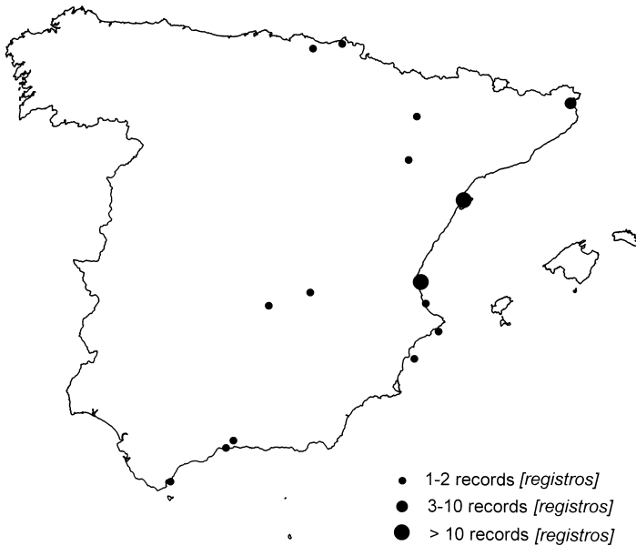
FIG. 1.—Distribution of the Aquatic Warbler Acrocephalus paludicola records in Spain during the spring migration (1965-1998). Due to scale restrictions, Canary Islands (two records) are not represented in the map. [Distribución de los registros de Carricerín Cejudo Acrocephalus paludicola en España durante la migración primaveral (1965-1998). Debido a restricciones de escala, las islas Canarias (con dos registros) no se representan en el mapa.]
