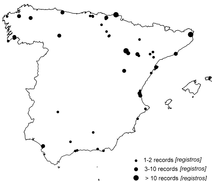
FIG. 2.—Distribution of the Aquatic Warbler Acrocephalus paludicola records in Spain during the autumn migration (1965-1998). Due to scale restrictions, Canary Islands (two records) are not represented in the map. [ Distribución de los registros de Carricerín Cejudo Acrocephalus paludicola en España durante la migración otoñal (1965-1998). Debido a restricciones de escala, las islas Canarias (con dos registros) no se representan en el mapa. ]
