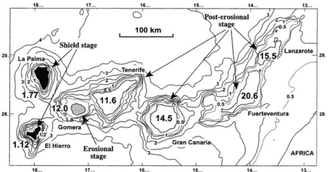
FIG. 1.—Oldest ages of subaerial volcanism in the Canary Islands (after Carracedo et al. , 2002). [Edades más antiguas de vulcanismo subaéreo en las islas Canarias (según Carracedo et al. , 2002).]
